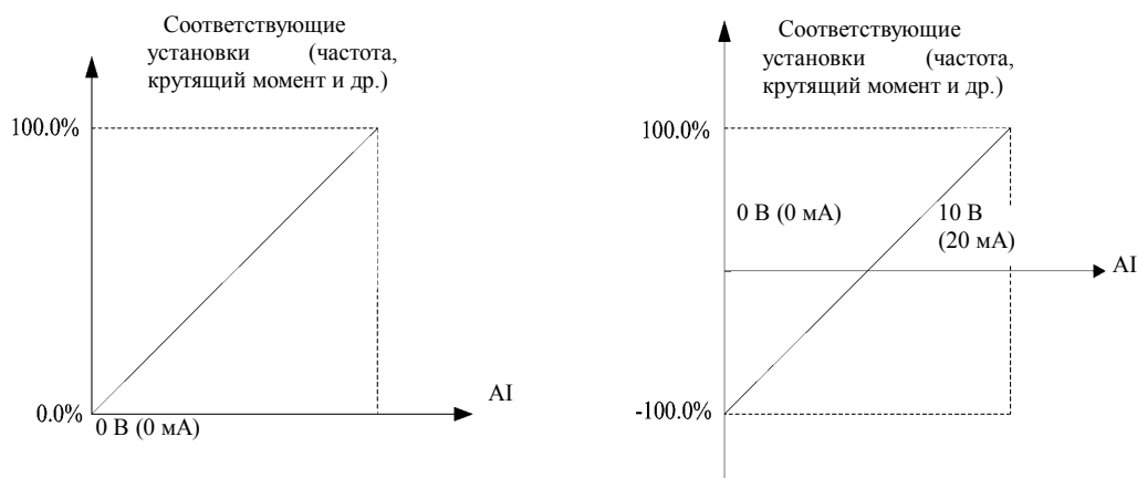
Рисунок 5-11. Соответствующее взаимоотношение между аналоговым опорным сигналом и установкой
